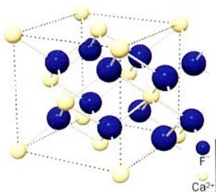
RED CRISTALINA DE FLUORURO DE CALCIO
