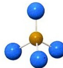
MOLÉCULA DE TETRACLORURO DE CARBONO
